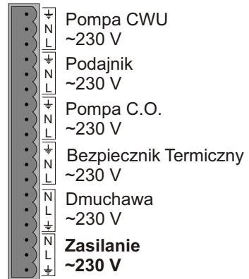
Listwa zasilania ~230V
